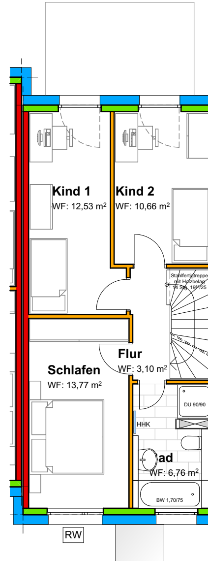
Obergeschoss
