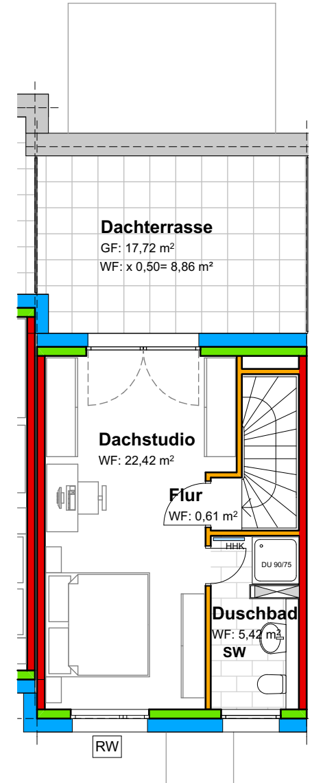
Dachgeschoss
